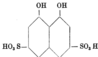
Chromotropsäure (siehe Tabelle S. 57).
